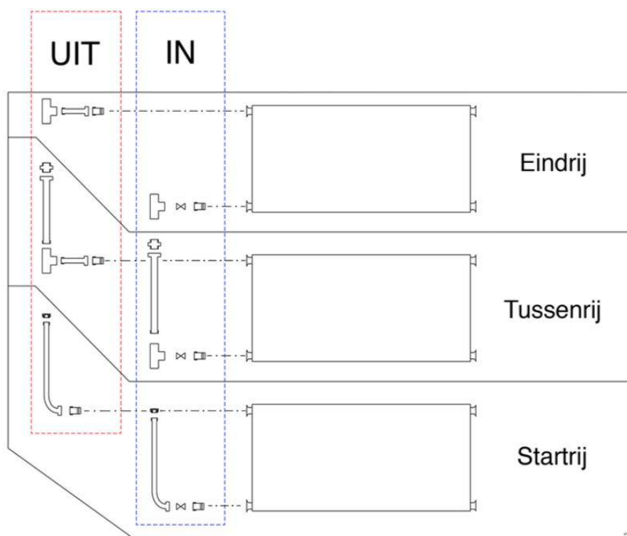
hydraulisch schema schuindak slangenpakketten
