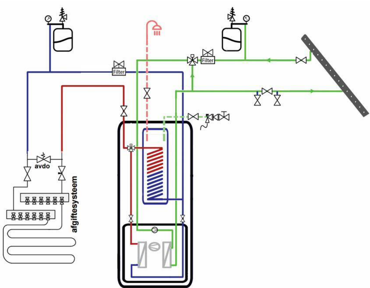
algemeen hydraulisch aansluitschema van het Triple Solar systeem
