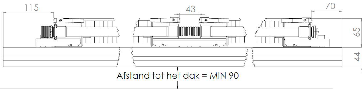
schuindak afdekplaat voor over het leidingwerk
