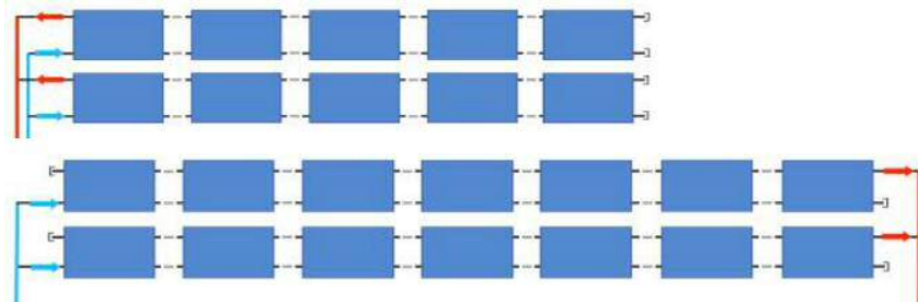
Bovenste figuur éénzijdige aansluiting, onderste figuur Tichelmann aansluiting
